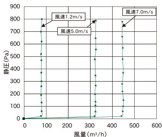
定風量特性 (φ 150)
