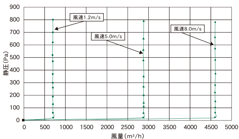
定風量特性 (400×400)
