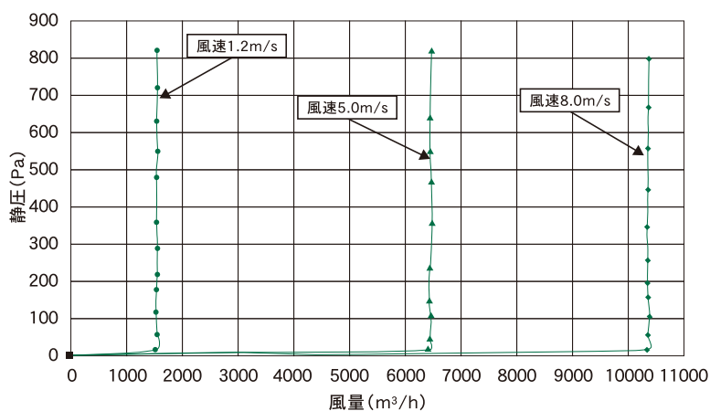
定風量特性 (600×600)
